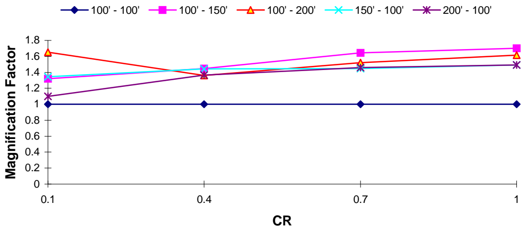
DOF 2 Magnification Factor : El Centro EQ T_1 = 0.5 s, T_R = 0.1
