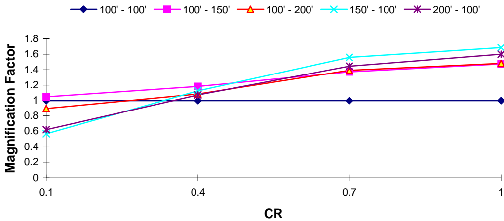
DOF 1 Magnification Factor : El Centro EQ T_1 = 0.5 \text{ s} , T_R = 0.1
