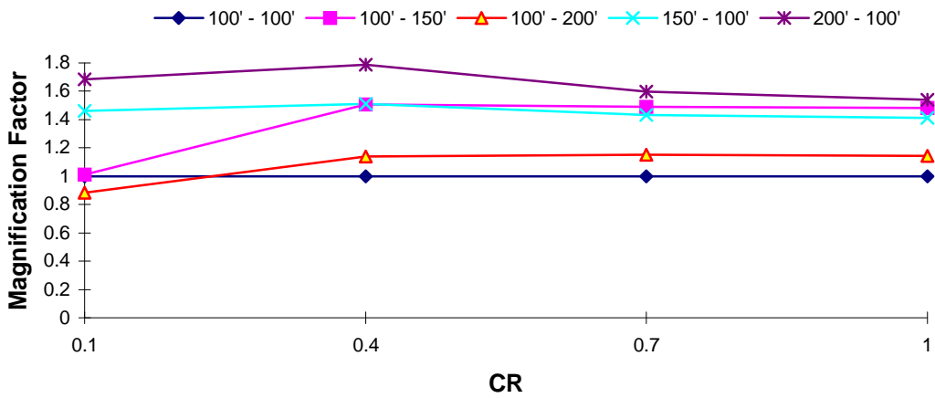
DOF 1 Magnification Factor : El Centro EQ T_1 = 1.5 s, T_R = 0.4
