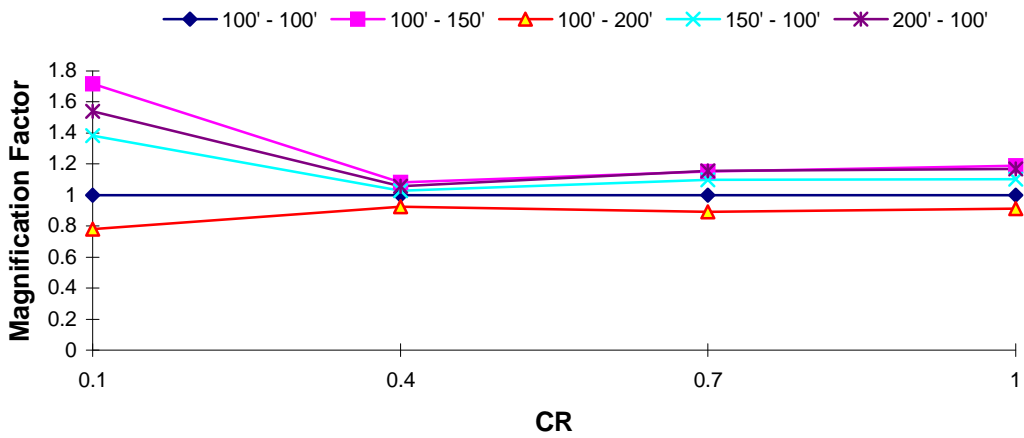
DOF 2 Magnification Factor : El Centro EQ T_1 = 1.5 \text{ s} , T_R = 0.7
