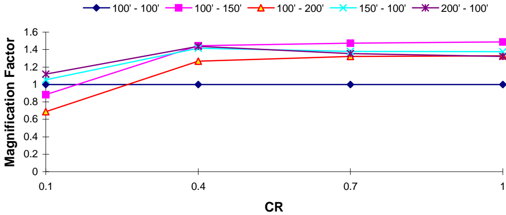
DOF 2 Magnification Factor : El Centro EQ T_1 = 1.5 s, T_R = 0.4
