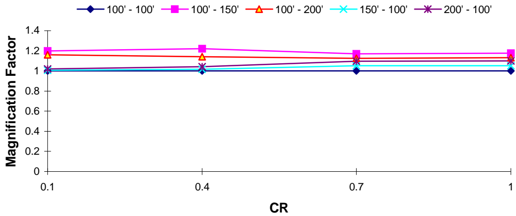
DOF 2 Magnification Factor : El Centro EQ T_1 = 2.5 \text{ s} , TR = 0.7
