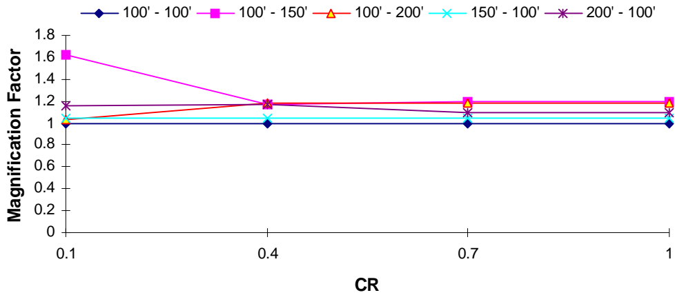
DOF 2 Magnification Factor : El Centro EQ T_1 = 3.0 s, T_R = 0.4
